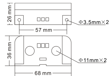
电流传感器(ETC100)
